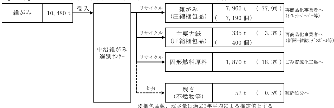
【参考】図3-10 令和4年度 中沼雑がみ選別センター 事業計画フロー図
