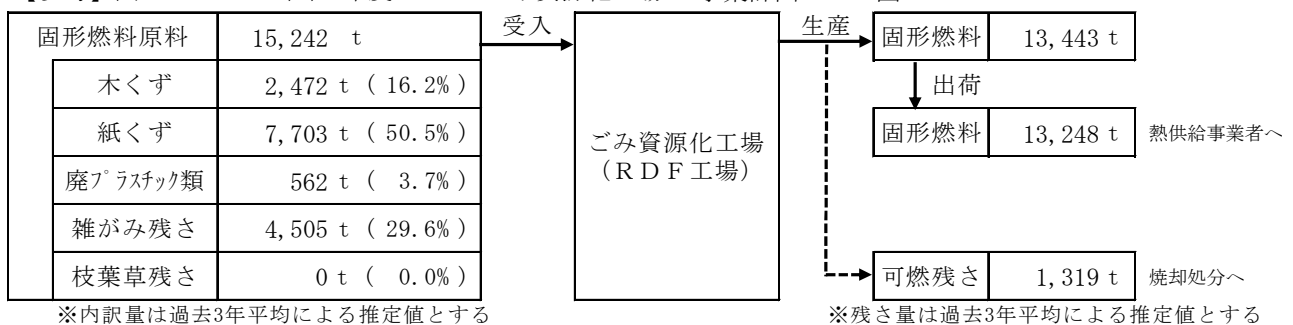
【参考】図3-6 令和4年度 篠路破砕工場 事業計画フロー図
